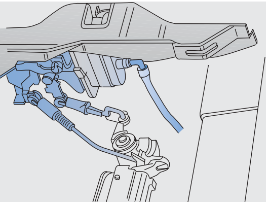
Stellmotor- Zentralverriegelung/ Tür links und rechts
